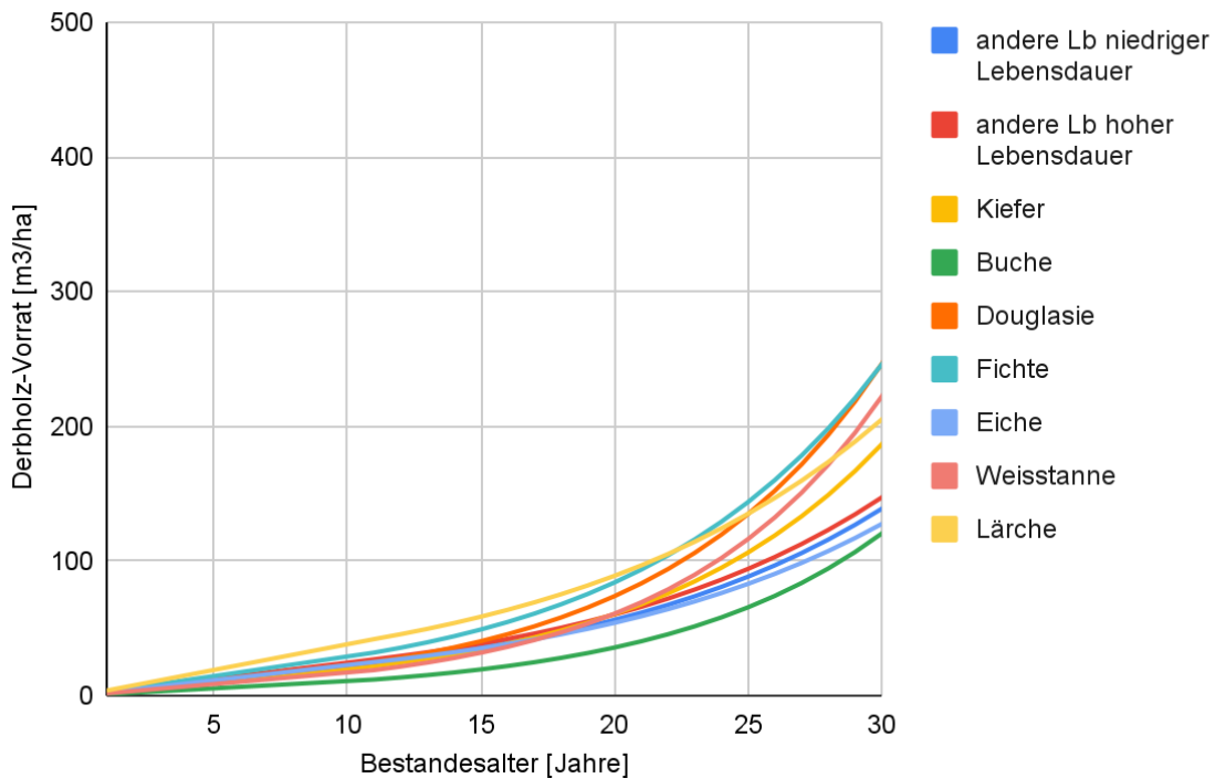
Abbildung 2: Entwicklung des Derbholz-Vorrates als Funktion des Bestandesalters nach dem dreistufigen Wachstum-Modells.
