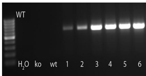
WT-PCR
